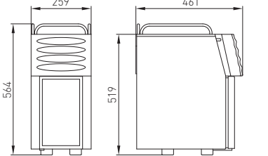
Beistellkühlleinheit
