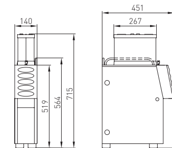
Pulversystem
